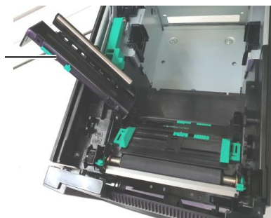
Sestav zgornjega tipala
