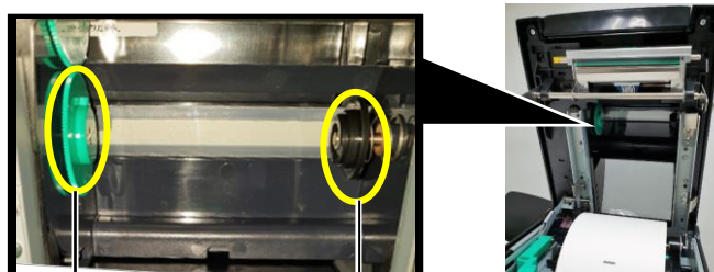
Uchwyt rolki (strona podawania)
