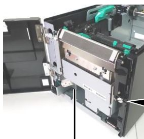
Moduł noża
