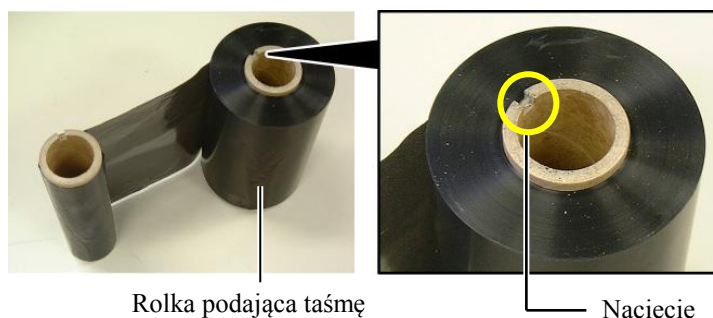
Uchwyt rolki (strona podawania)
