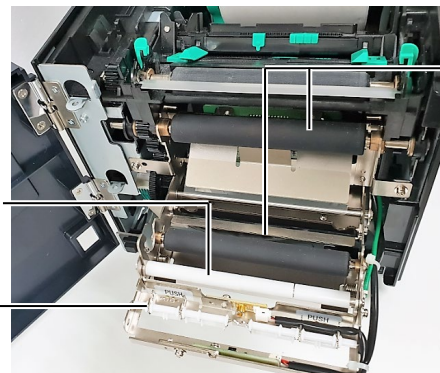
Guide Roller
