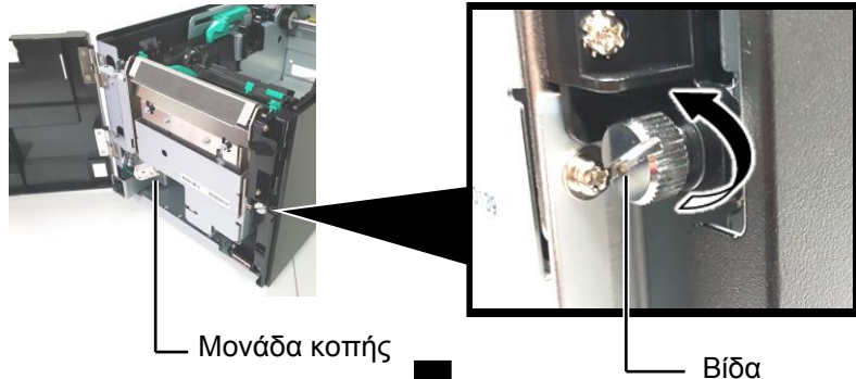
Μονάδα κοπής
