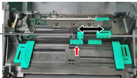
間隙探測器
