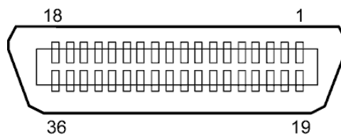
Anslutning IEEE1284-B
