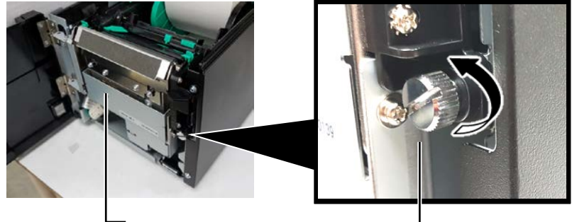
고정 나사
