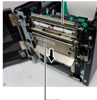
해제 바
