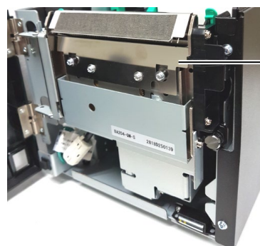
Exterior de la cuchilla del cortador
