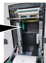
Soporte de cinta (lado de suministro)
