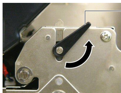
Piespiedruļļa svira
