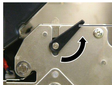
Piespiedruļļa svira
