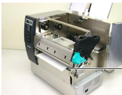
Materiāla izvads
