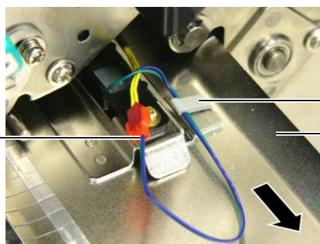
Kabeļu klipšis
