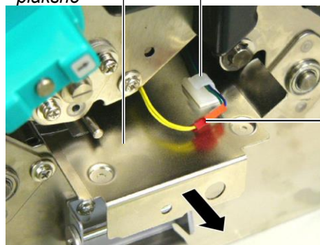
Materiāla vadotnes plāksne
