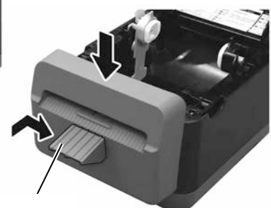
Vágótálca
