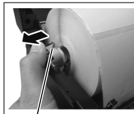
Μοχλός θήκης ρολού χαρτιού
