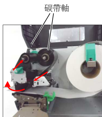
外卷碳帶
