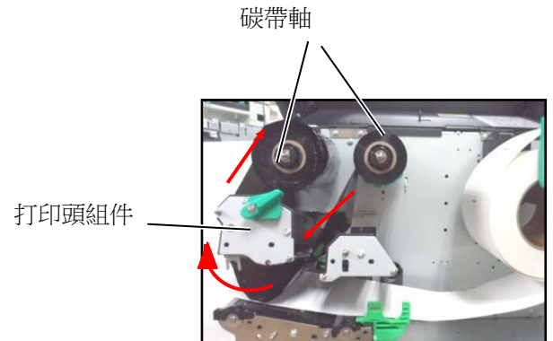
內卷碳帶
