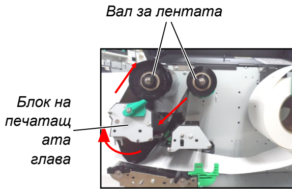
Лента, която се навива навътре
