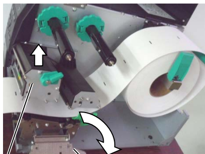
Блок на печатащата глава
