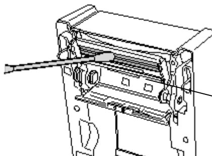
Elementul capului de imprimare (poziționat la marginea capului de imprimare)
