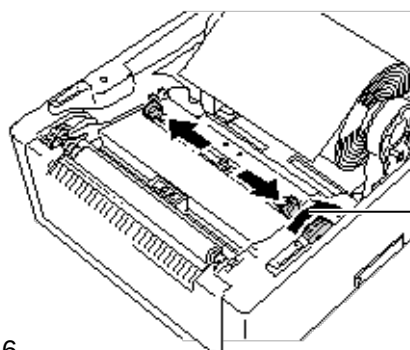
Disc de reglare a ghidajului pentru suport
